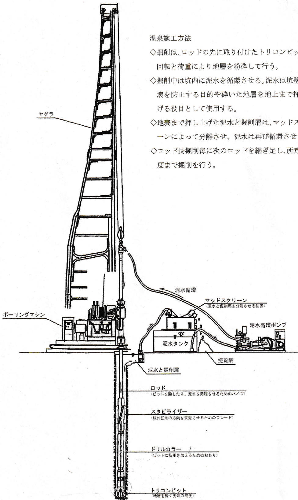
ボーリング施工立面図
